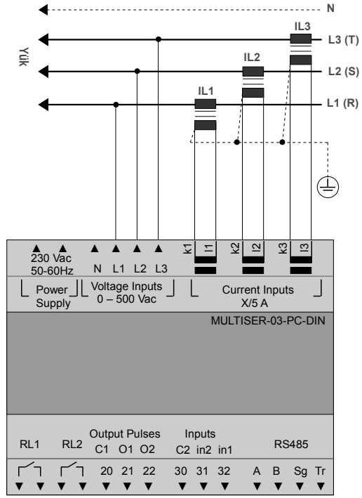
3 Faz Nötrsız Bağlantı
