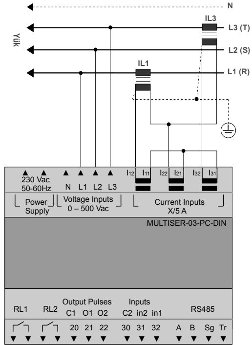
3 Faz Nötrsız ARON Bağlantı
